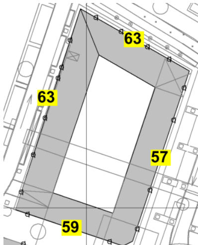
Figuur 5.3: Gecumuleerde geluidbelasting op basis van wegverkeerspectrum
