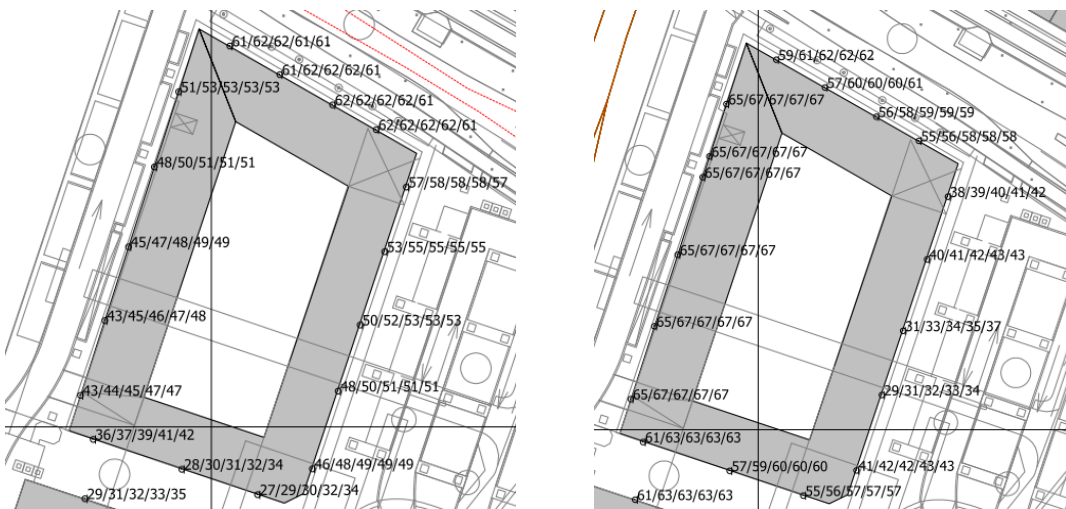
Figuur 5.2: Geluidbelasting ten gevolge van wegverkeer (links) en ten gevolge van railverkeer (rechts)
